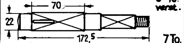
Gewindezapfen Raccord filté ab 5* t verstärkt 4-Kant 18mm
