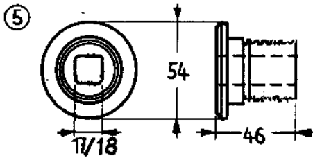
Gewindezapfen Raccord filté ab 5* t verstärkt 4-Kant 18mm
