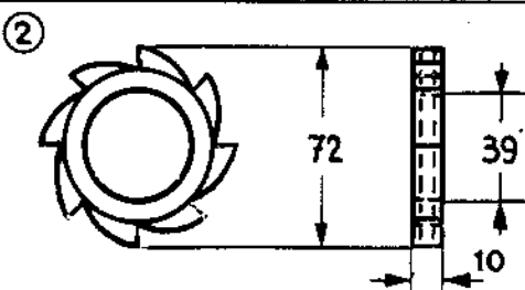
Sperrad roue à rochet
