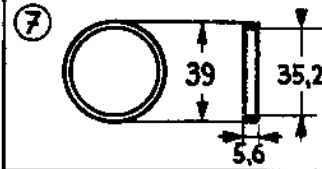
Laufring Bague en plast.
